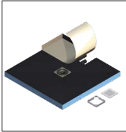
Komplettboard E65 Ablauf mittig BA E65 (Board mit waagerechtem Ablauf und Ablaufabdeckung E65) Gesamteinbauhöhe nur 65 mm!
