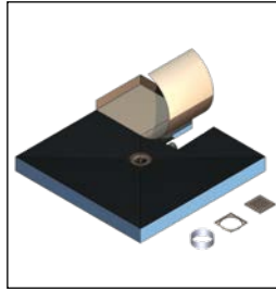
Komplettboard E90 Ablauf mittig BA E90 (Board mit waagerechtem Ablauf und Ablaufabdeckung E90) Gesamteinbauhöhe nur 90 mm bei normkonformer Sperrwasserhöhe!
